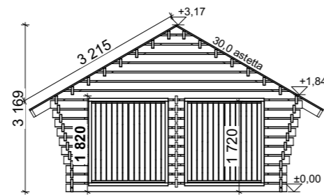
Snitt 1:100
