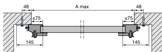
Asennus lisävarusteena saatavalla erikoisankkurilla autotallin sivuseinään
