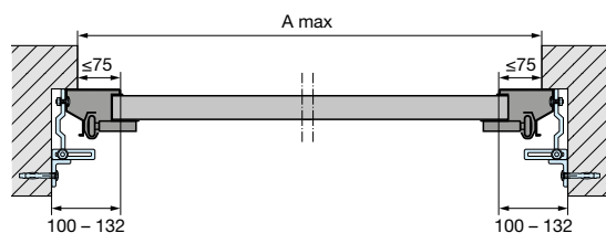
Asennus lisävarusteena saatavalla erikoisankkurilla autotallin sivuseinään
