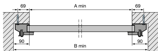
Asennus lisävarusteena saatavalla kulma-ankkurilla
