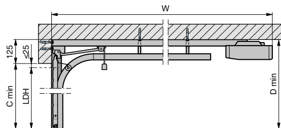
Leikkaus pystysuunnassa
