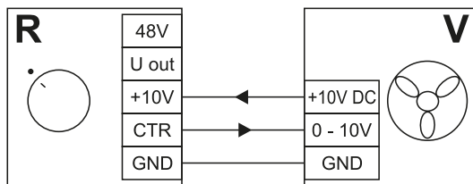
Kytentäkaavio
