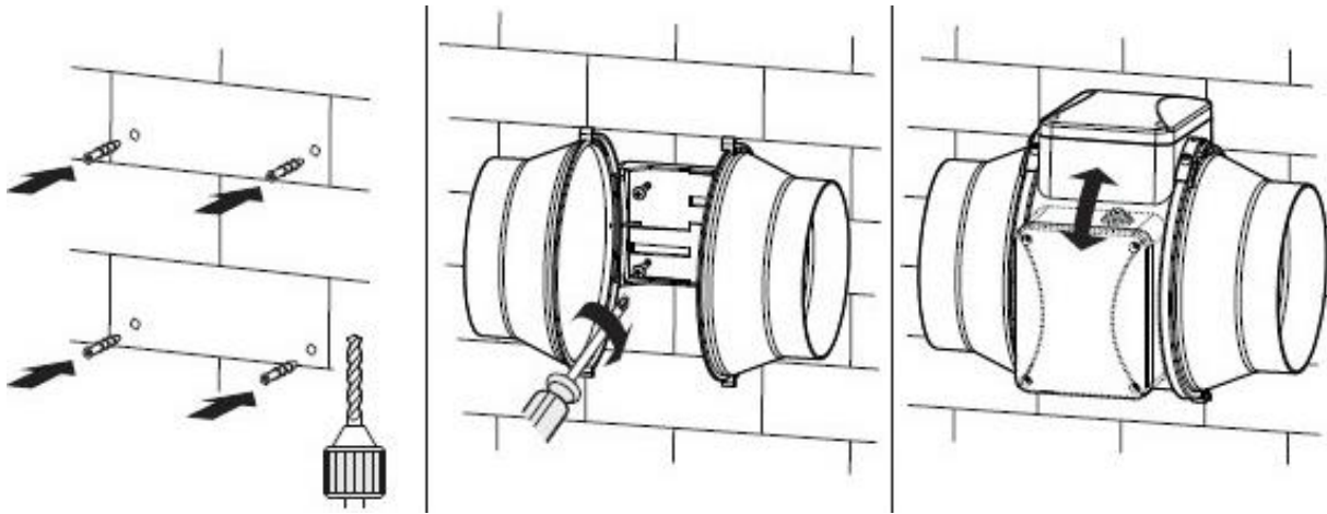
Kuva 7: Pora reiät, asenna kiinnitysankkurit ja kiinnitä puhallin sekä moottori takaisin paikalleen
