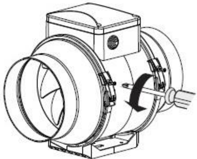
Kuva 10: Irrota moottorin kiinnitysruuvit
