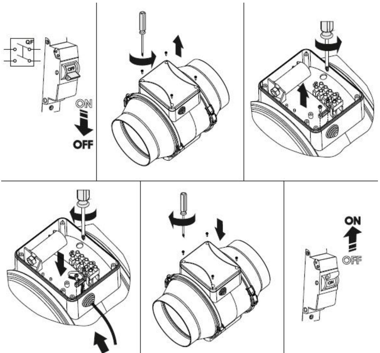
Kuva 8: Katkaise virta, irrota sähkökytkentärasian kansi, kytke virtajohto kytkentäkaavion mukaisesti ja kiinnitä kansi uudelleen ja laita lopuksi virta takaisin päälle.
