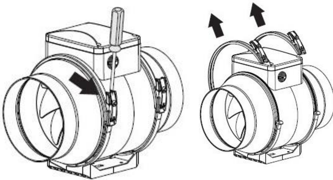
Kuva 5: Irrota moottorin kiinnitysruuvit ja poista moottori ylöspäin nostamalla
