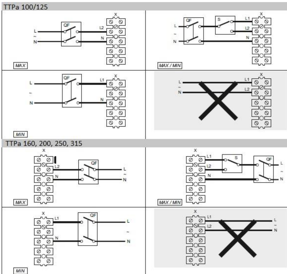
Kuva 12: Kytkentäkaavio
