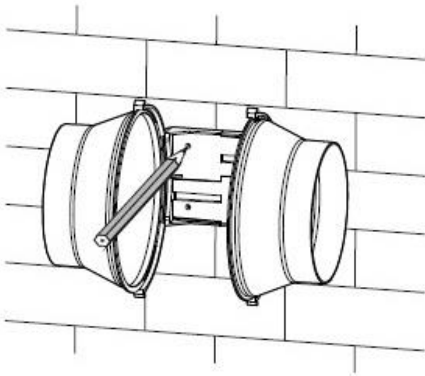
Kuva 6: Merkkää kiinnitysreiät esim. lyijykynällä seinään/kattoon
