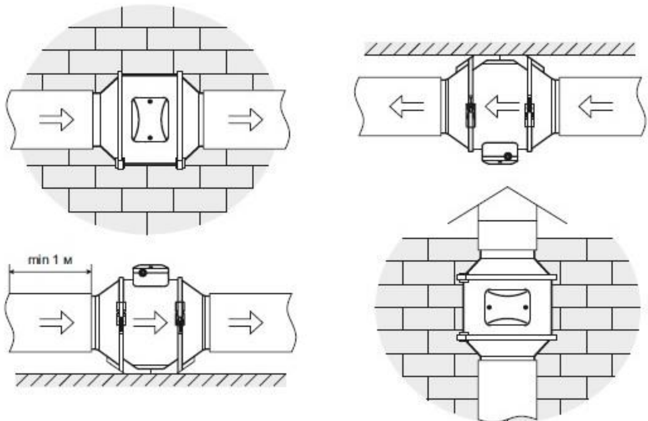
Kuva 1: Puhaltimen asennus
