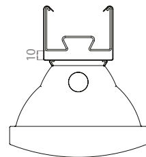
AMJK2 asennus
