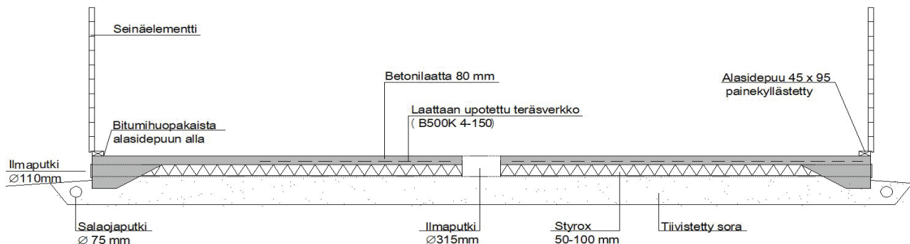
Perustukset Leikkaus A - A:
