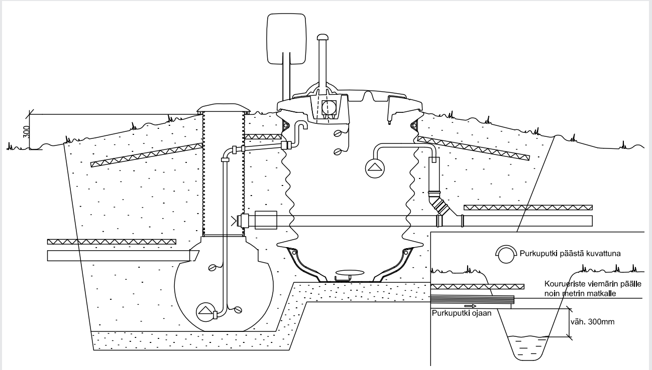
Kuva 23: Maakummun asennus
