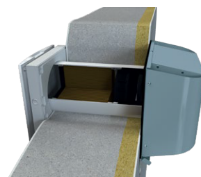
Asennusesimerkki ohuille seinille. AH-S grey 160 / AH-S chrome 160
