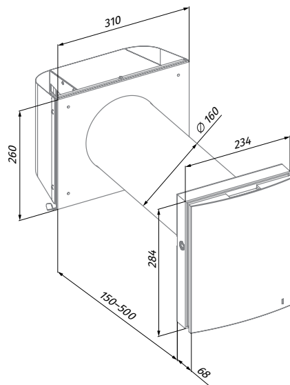
Vento Expert A50-1 S Pro (ohuille seinille)
