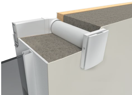
Kulma-asennus seinän sisälle KIT BlauPlast white 160 / KIT BlauPlast chrome 160
