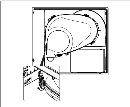
Kuva 10.36 Imutilan kiinnikkeet
