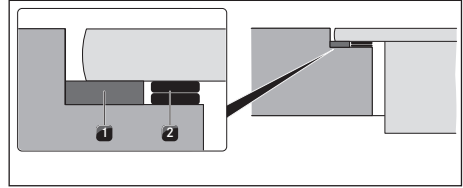
Kuva 10.15 Korkeussäätölevyt
