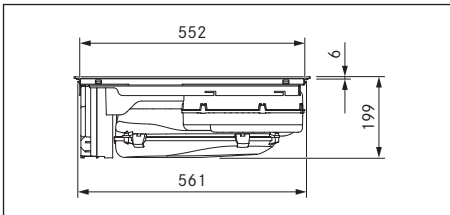
Kuva 3.5 Laitemitat PURSU kuva edestä
