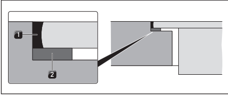
Kuva 10.25 Tiivistenauha uppoasennuksessa
