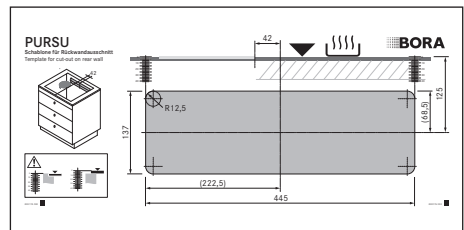
Kuva 10.22 Sapluna takaseinän aukkoa varten
