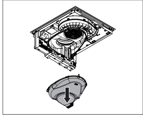
Kuva 10.37 Imutilan alaosan irrottaminen
