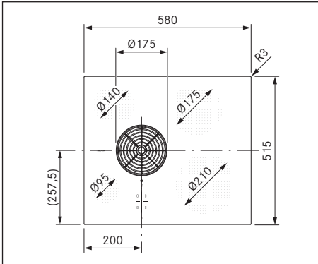
Kuva 3.4 Laitemitat PURSU kuva ylhäältä
