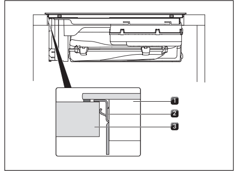
Kuva 10.27 Keittotason kiinnittäminen
