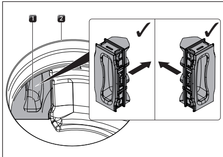
Kuva 8.10 Suodattimen vaihtoläpän asettaminen
