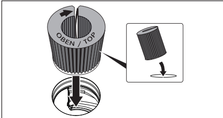
Kuva 10.33 Aktiivihiilisuodattimen asettaminen tuloaukkoon
