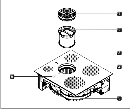
Kuva 5.1 Keittotas
