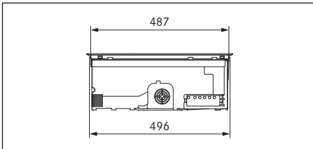
Kuva 3.6 Laitemitat PURSU sivukuva
