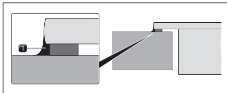
Kuva 10.47 Silikonitiivistysmassa pinta-asennuksessa
