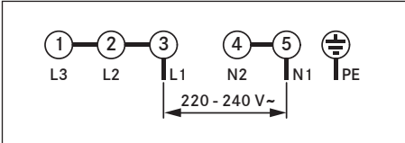
Kuva 10.40 Liitäntäkaavio – 1-vaiheiliitäntä
