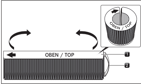
Kuva 10.32 Aktiivihiilisuodatin
