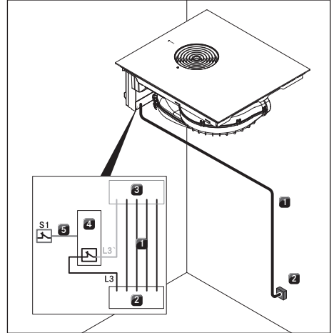
Kuva 10.42 Liitäntäkaavio, ulkoinen kytkin
