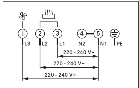
Kuva 10.38 Liitäntäkaavio - 3-vaiheiliitäntä
