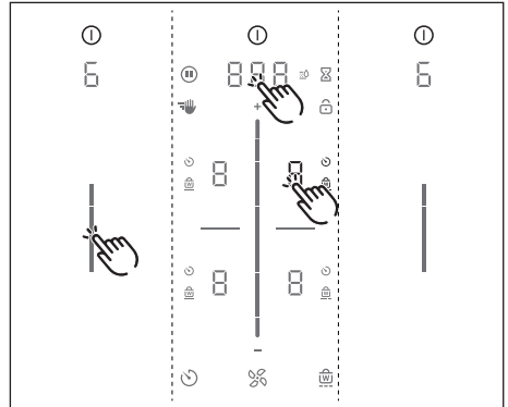
Kuva 7.6 Valikkokohta 6: LED-testi
