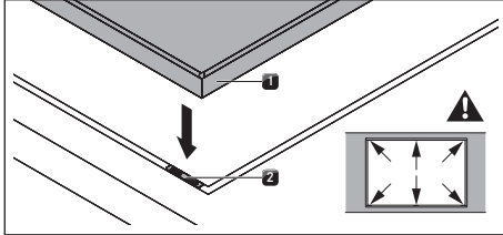
Kuva 10.28 Korkeussäätölevyt
