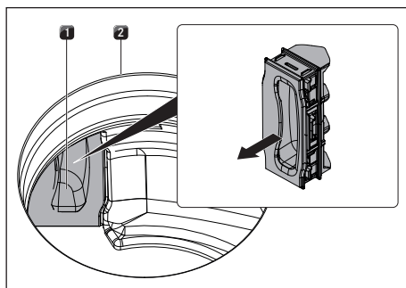
Kuva 8.4 Suodattimen vaihtoläppän irrottaminen
