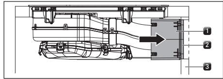
Kuva 10.30 Takaseinän liittäminen
