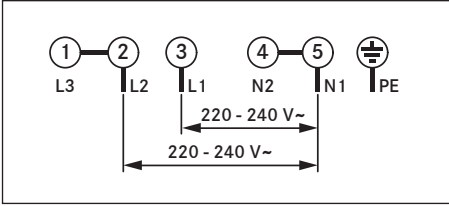
Kuva 10.39 Liitäntäkaavio – 2-vaiheiliitäntä
