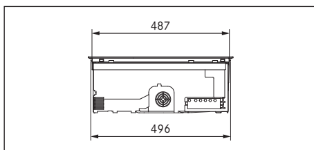
Kuva 3.3 Laitemitat PURSA sivukuva
