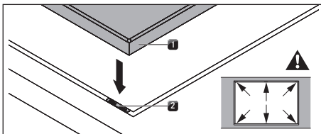
Kuva 10.14 Korkeussäätölevyjen asettaminen
