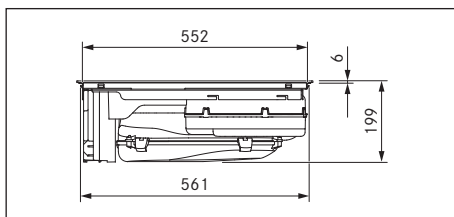
Kuva 3.2 Laitemitat PURSA kuva edestä
