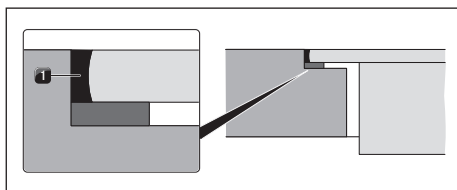
Kuva 10.48 Silikonitiivistysmassa oppoasennuksessa
