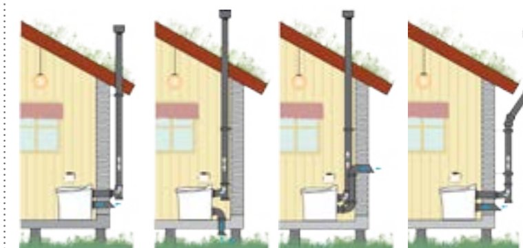
COMFORT-käymälän asennus
