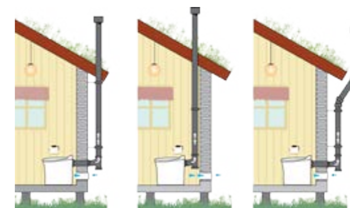
CLASSIC-käymälän asennus
