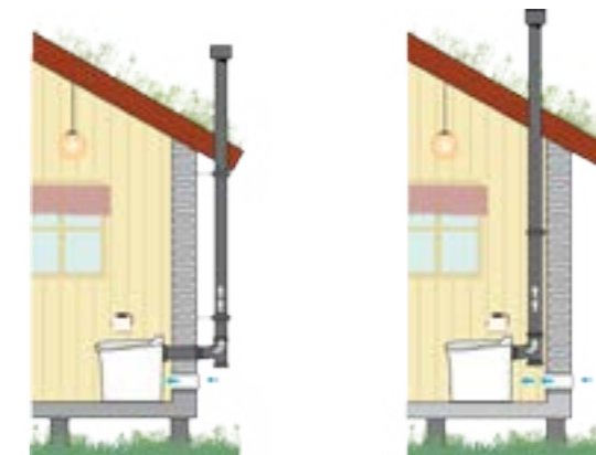
GAS-käymälän asennus
