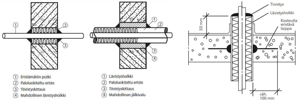
Esimerkki putken viemisestä betoniseinän läpi.
