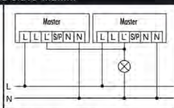
Kork, 6 laitteen rinnankytkentä
