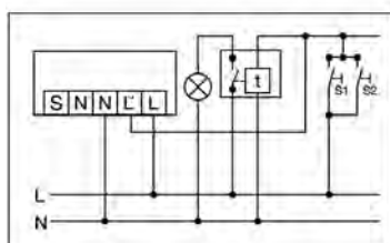
Rinnankytkentä porraskäytävävalaistusautomaatin kanssa.
