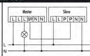
Master-Slave-kytkentä (korkeintaan 10 Slave-laitetta voidaan liittää yhteen Master-laitteeseen).
