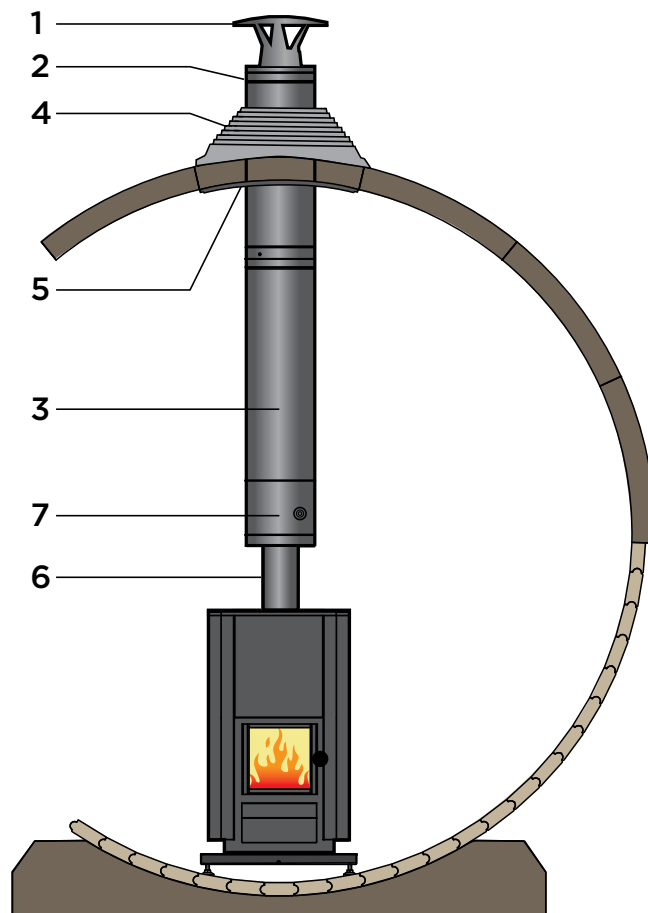
Esimerkki tynnyrisaunan piippukokonaisuudesta
