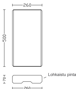
HB-ISOKansikivi
