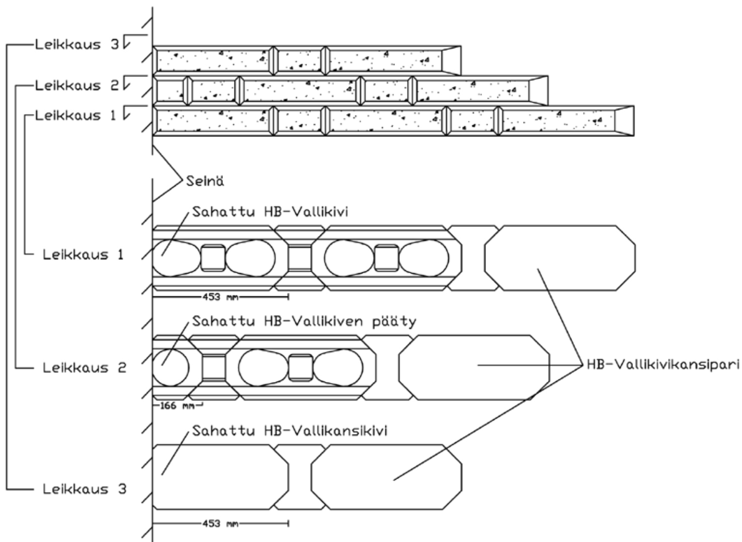
Kuva 11. Aloitus seinästä.
