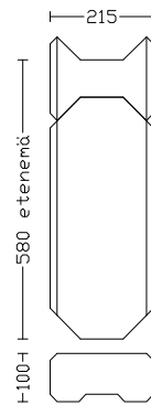
HB-ISOKansikivi
