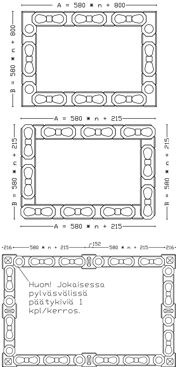
Kuva 17. Kukka-allasmalleja.
