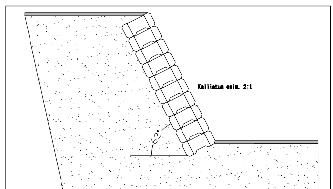
Kuva 12. Kallistettu muuri.
