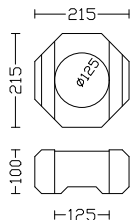
HB-Päätykivi
