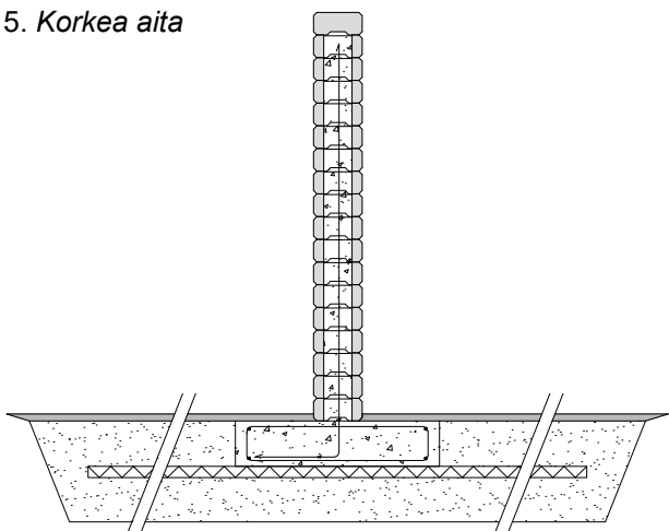
Kuva 2. Matala muuri
