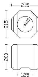
HB-ISOPäätykivi
