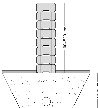
Kuva 3. Matala aita
