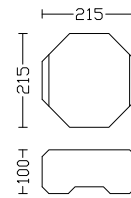
HB-Kansipäätykivi
