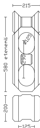
Kuva 1. HB-Vallikivi-tuoteperhe
