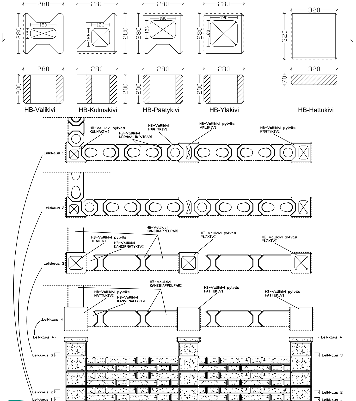
Kuva 13. HB-Pylväskivet ja pylväskivien käyttöperiaatteet.
