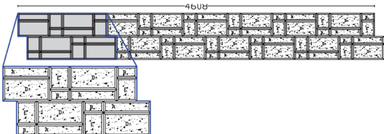
Kuva 16. Sekoiteseinän esimerkkiladonta.
