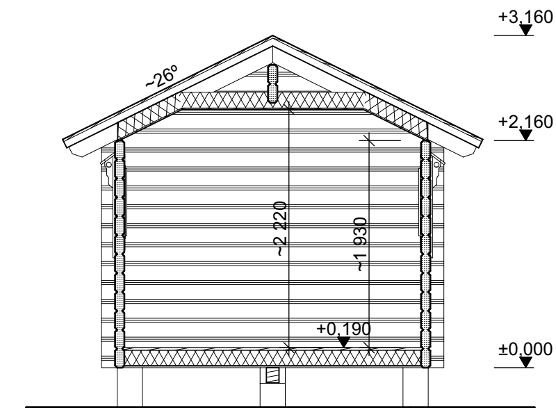
LEIKKAUS A - A 1:50
