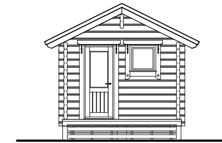
JULKISIVU 1 1:100
