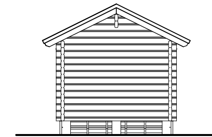
JULKISIVU 3 1:100
