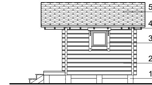
JULKISIVU 4 1:100
