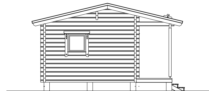
JULKISIVU 2 1:100
