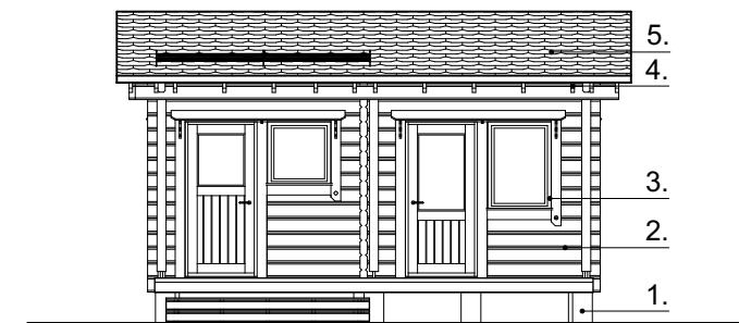
JULKISIVU 1 1:100
