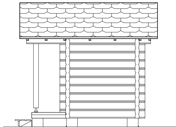
JULKISIVU 4 1:50
