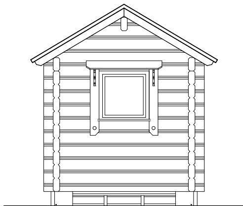
JULKISIVU 3 1:50
