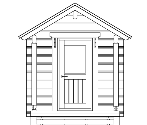
JULKISIVU 1 1:50
