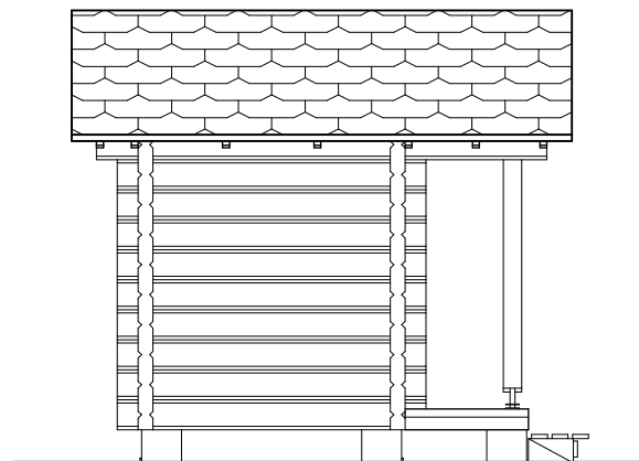
JULKISIVU 2 1:50
