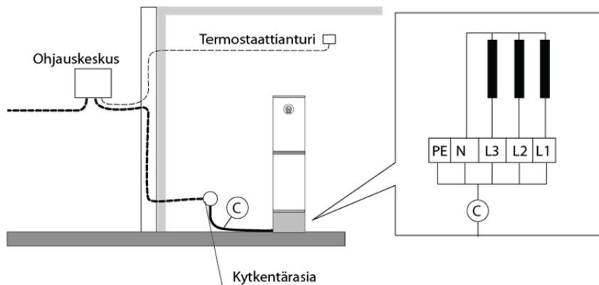
Kiukaan sähkökytkentä 2-syöttö
