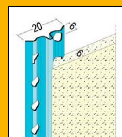
Rappausohjuri
