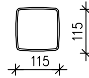
Menekki 76kpl/m 2 KLASSIKKO NELIÖKIVI
