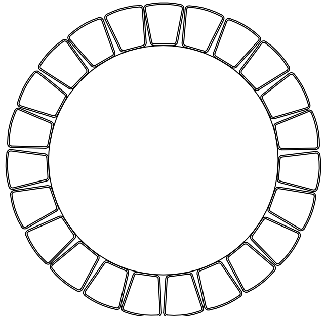
Ø 600, 23 KPL KLASSIKKO KAARREKIVIÄ
