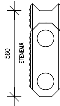
LOHKOMUURIKIVIPARI Menekki 17,8 kiviparia/m 2
