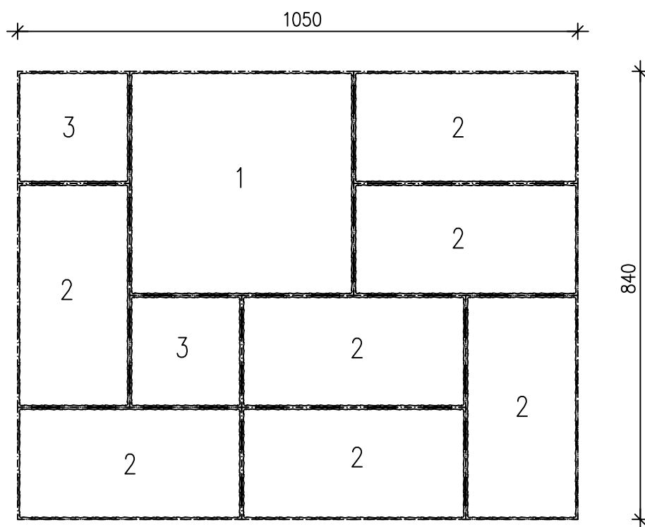
VALMIS LADONTAKUVIO LAVAKERROKSISSA 0,88 m 2
