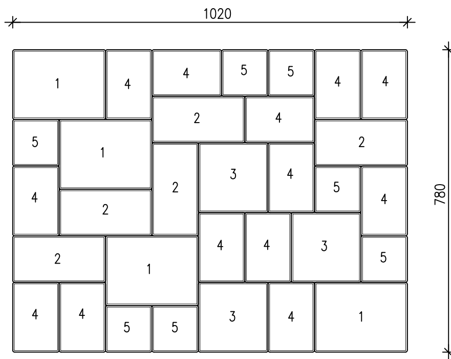
VALMIS LADONTAKUVIO LAVAKERROKSISSA 0,8 m 2
