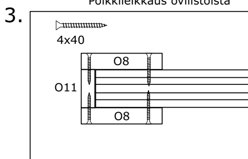
Poikkileikkaus ovilistoista
