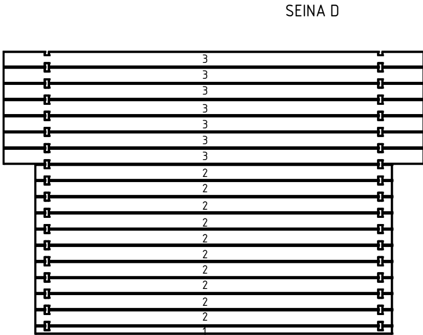
Otsa- ja räystäslautojen asennuskuva
