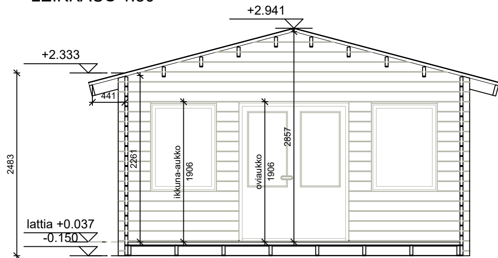
LEIKKAUS 1:50
