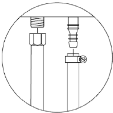
Painesäätimen letkun kiinnitys
