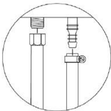
Fastsättning av tryckregulatornslang
