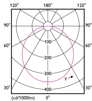
Downlight DN065B G2 LED10 830 D150 RD EU
