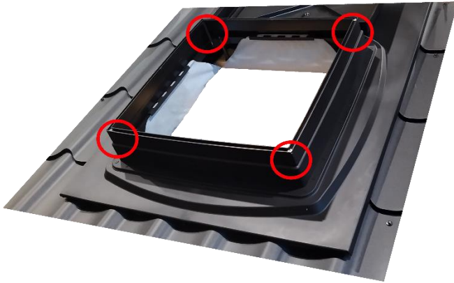
Kuva 8. Ruuvien paikat
