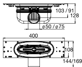
Poistoputki sivulle Ø50/75
