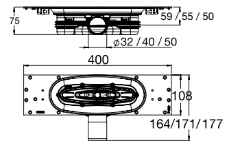
Matala poistoputki sivulle Ø32/40/50
