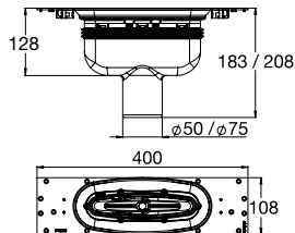
Poistoputki alas Ø50/75
