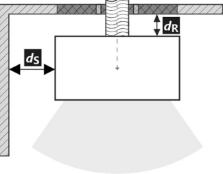
Hinterer Rauchrohranschluss
