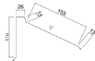
9. Pulpettikaton ylärästäslista, L = 3000 mm
