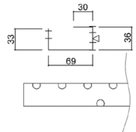
7. Harjantiivistelista, L = 460 mm, L=510 mm ja L = 3000 mm
