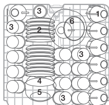
DW60M6050 DW60M6051 (14 platsinställningar)
