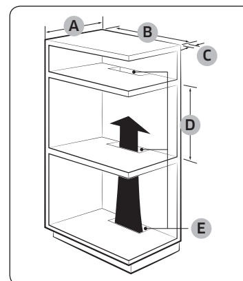
Indbygningsskab (mm)
