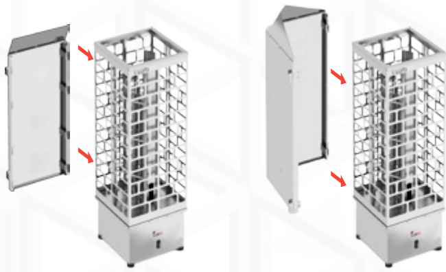
Seinäasennus erillisellä suojaseinällä
