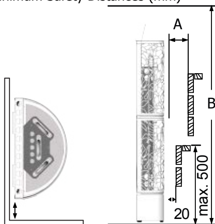
Kuva 2 Vähimmäisturvaetäisyydet (mm) Fig. 2 Minimum Safety Distances (mm)
