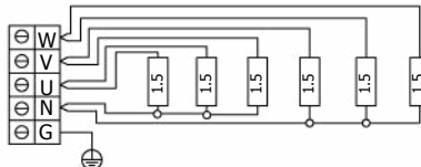
DRFT6-90NS-WL 9,0 kW
