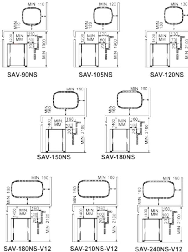
Kuva 2 | Vähimmäisetäisyydet (mm) Fig. 2 | Minimum safety distances (mm)
