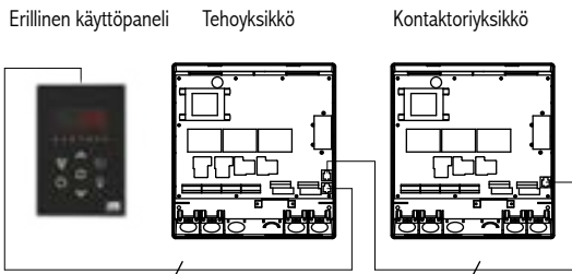
Kuva 4 Tehoyksikön, erillisen käyttöpaneelin ja kontaktoriyksikön asennus.
