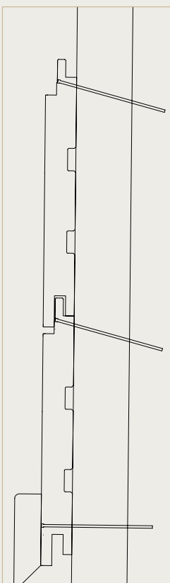
Esimerkki piilokiinnityksestä
