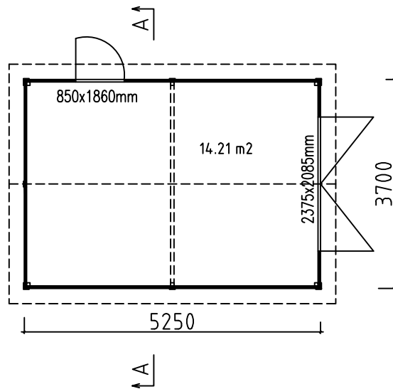
POHJAPIIRUSTUS
