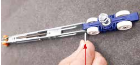
1. Yhdistä hidastin pyörästöön sokkatapilla.
