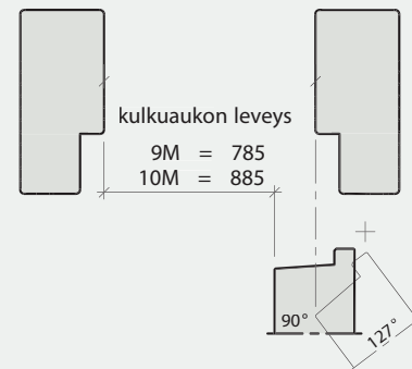
Oven avautuminen peruskarmilla
