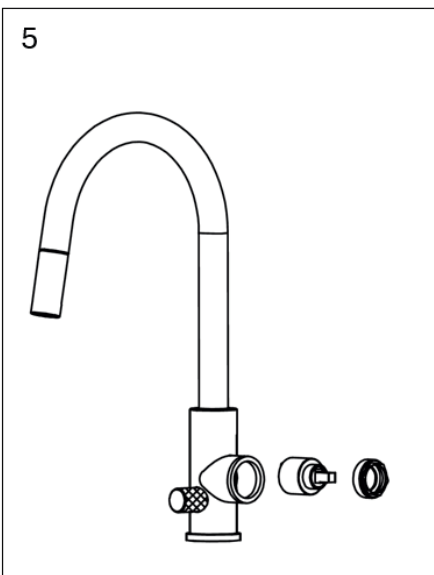
KUVA 5 | BILD 5 | IMAGE 5 FI Irrota mutteri ja poista säätöosa. Vaihda se uuteen ja kokoa osat takaisin päinvastaisessa järjestyksessä kuin purkaessa. SE Ta bort muttern och avlägsna patronen. Byt ut den mot en ny och montera tillbaka delarna i omvänd ordning. EN Remove the nut and take out the cartridge. Replace it with a new one, then reassemble all parts in the reverse order of removal.
