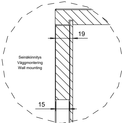
DET1 1:2
