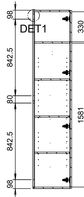
A-A
