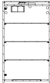
B-B
