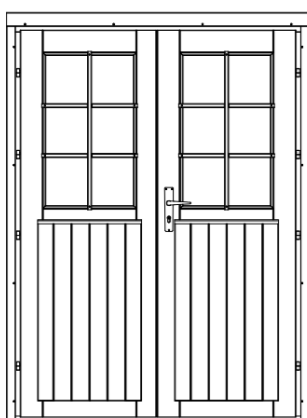
Doppeltür 70 mm ISO 1425 x 1955 mm 1 st.
