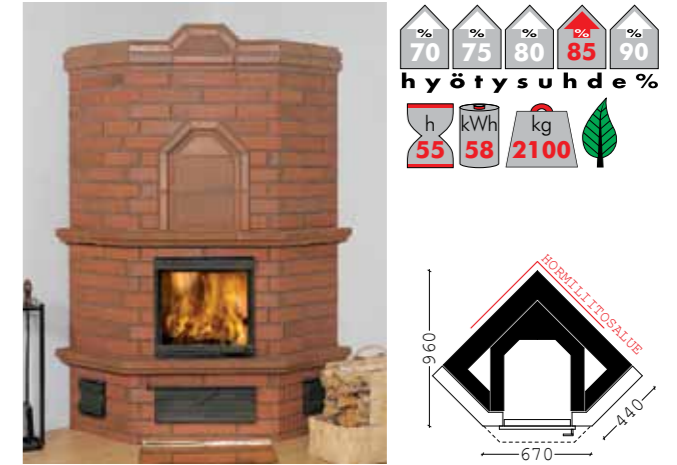
Kuori: Kaamos vaalea Antiikki Sauma: Ropis Luukku: Euro musta, valurauta Koristeet: Liekkivaalea
