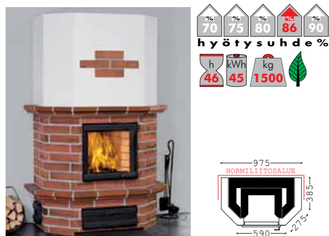
Yläosa: Antiikkilaasti, valkoinen Alaosa: Ruukintili "käsinlyöty", punaisenkirjava Sauma: Harmaa Luukku: Euro musta, valurauta
