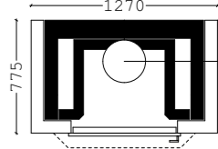
Väri: Antiikkilaasti, valkoinen Kaakeli: Hiili, lisähinta Luukku: Grafitti, teräs Puutila: Antiikkilaasti/hiilikaakeli
