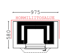
Face: Tummanharmaa kirjava Sivu: Valkoinen Luukku: Satiinikromi, teräs
