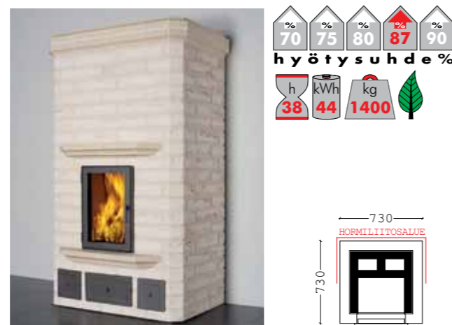
Kuori: Ruukintili vaalea "käsinlyöty" Sauma: Tundra Luukku: Grafiitti, teräs Koristeet: Fenix
