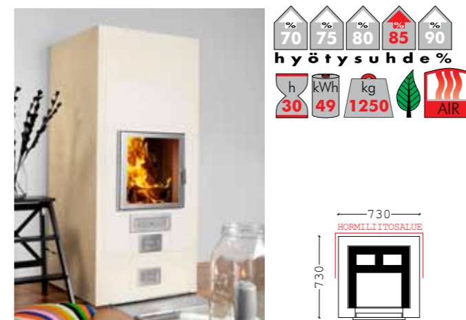
Väri: Vanilja Mosaikki: Luonnonvalkoinen Luukku: Satiinikromi, teräs
