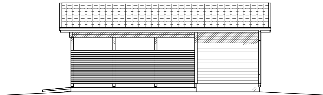
JULKISIVU 2.
