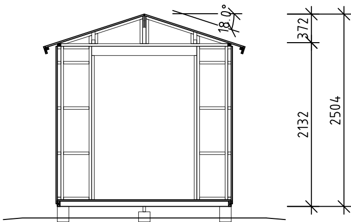
LÄPILEIKKAUS
