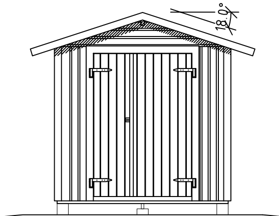
PÄÄTY, OIKEA
