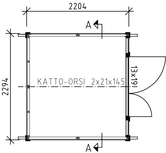
SUUNNITELMA
