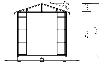
Läpileikkaus
