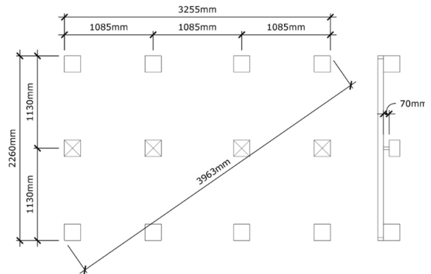
Perustuspiirustus
